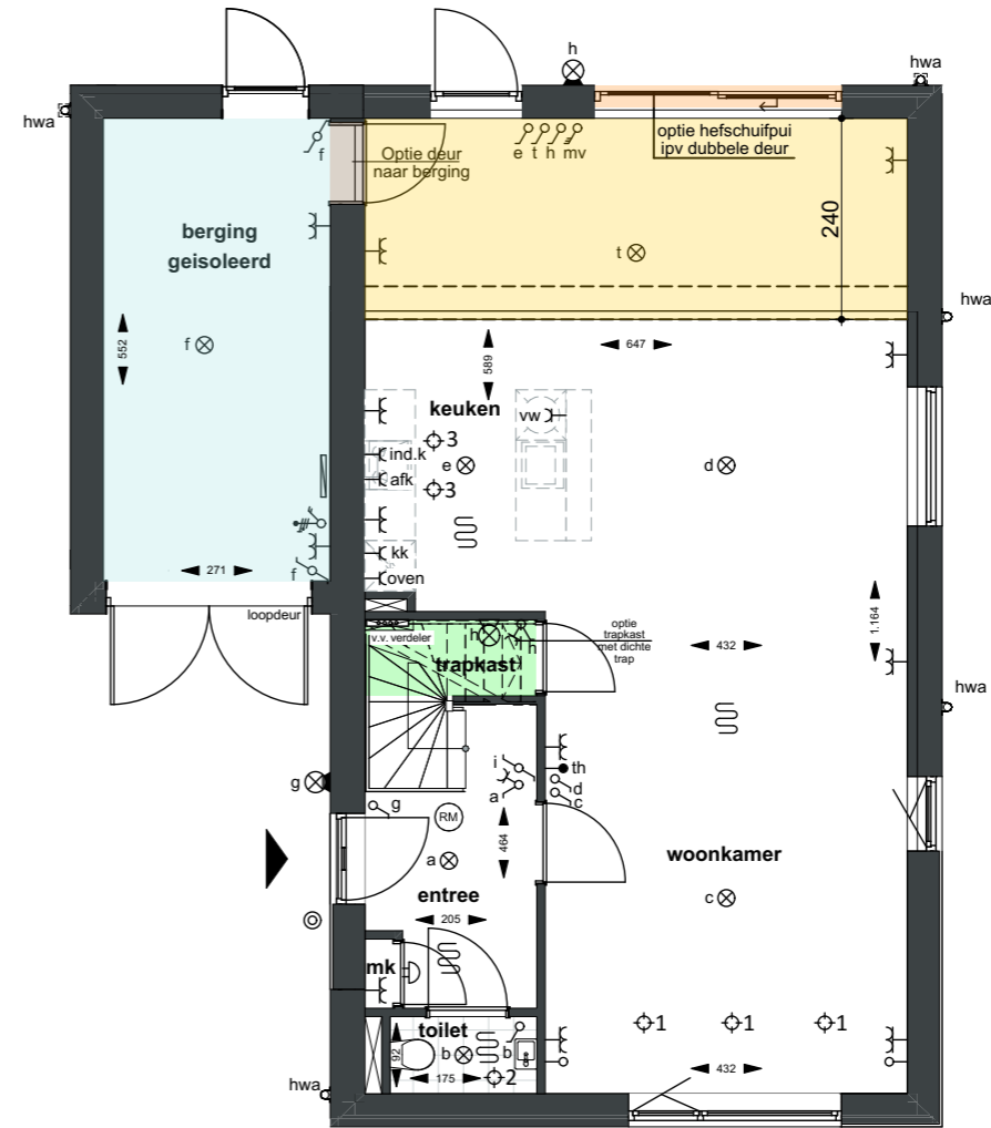
BEGANEGROND
