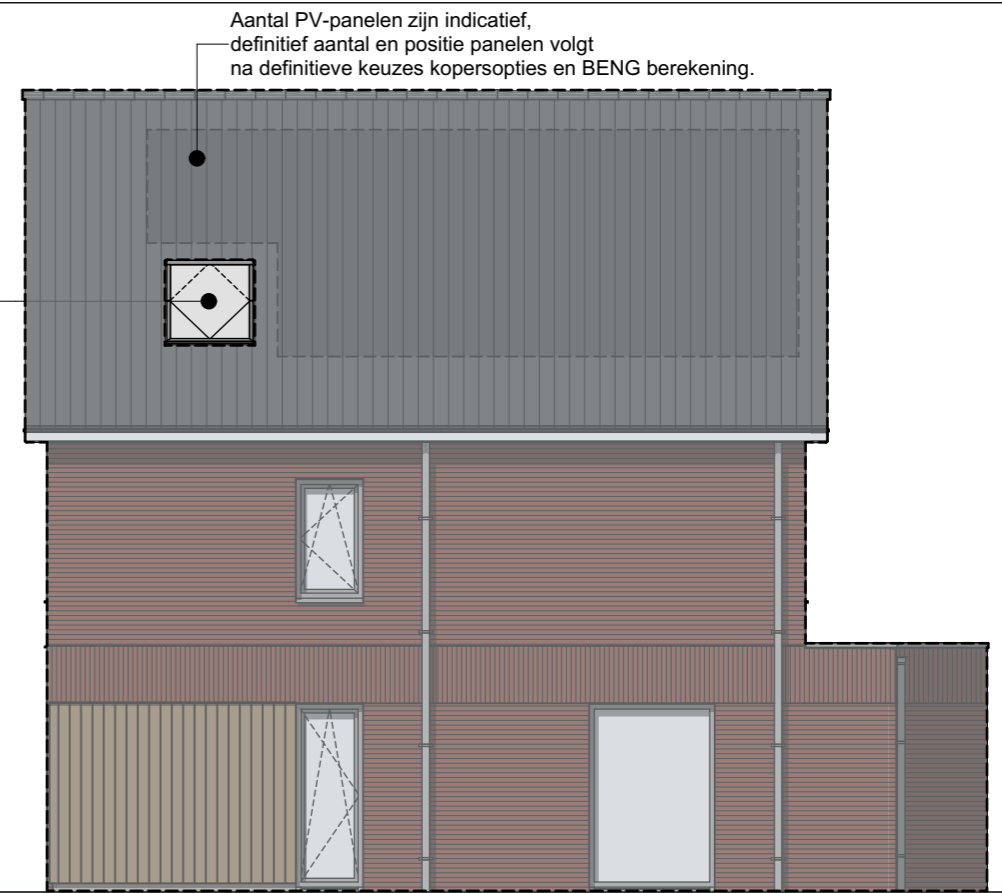
RECHTERGEVEL
