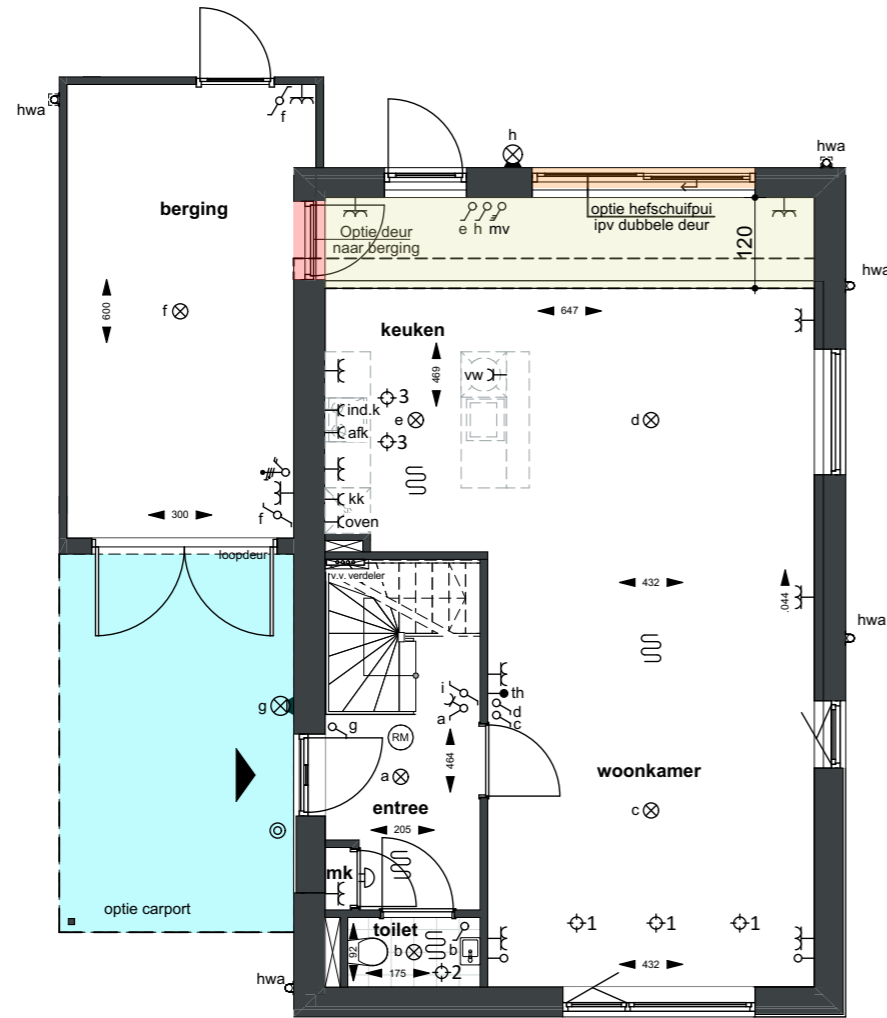
BEGANEGROND
