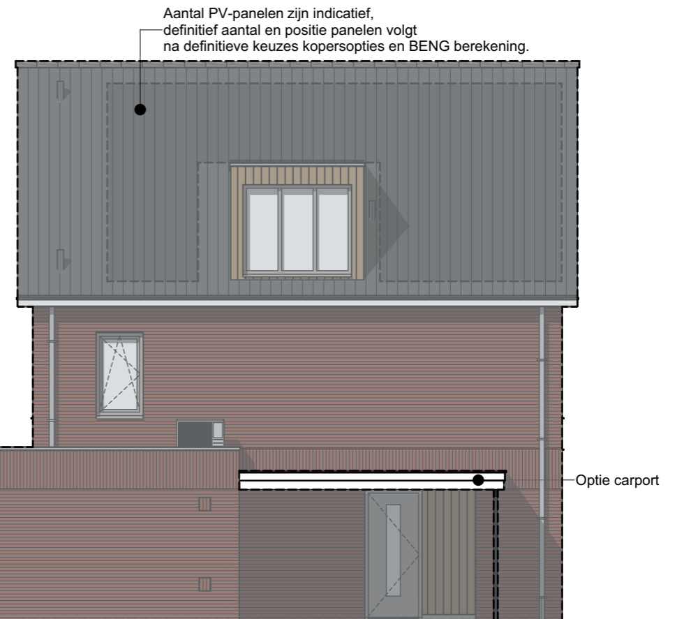
RECHTERGEVEL
