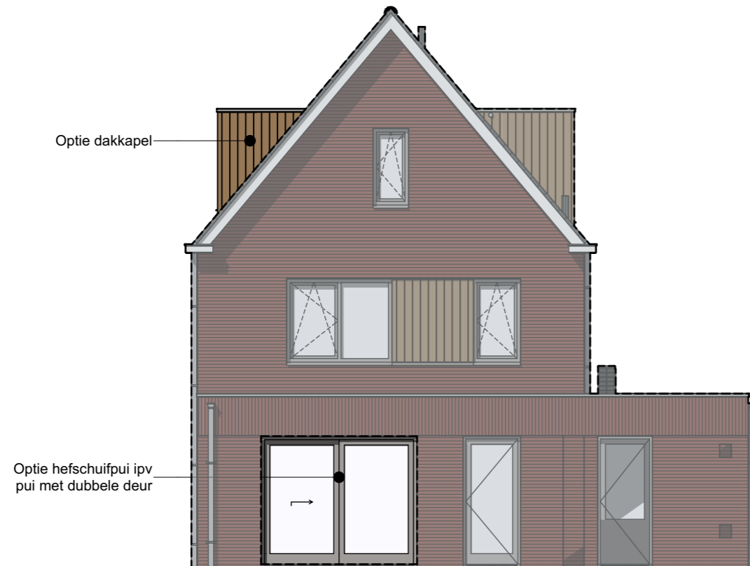
ACHTERGEVEL
