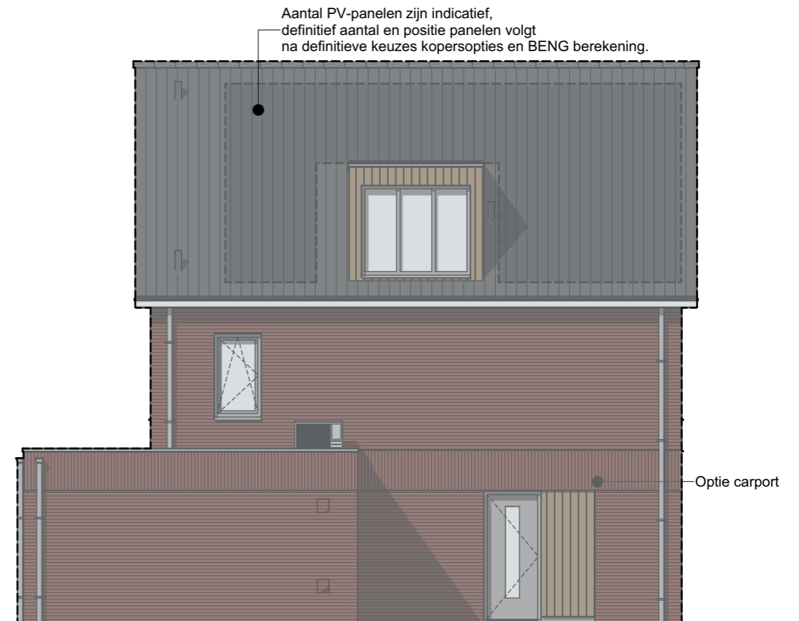
RECHTERGEVEL
