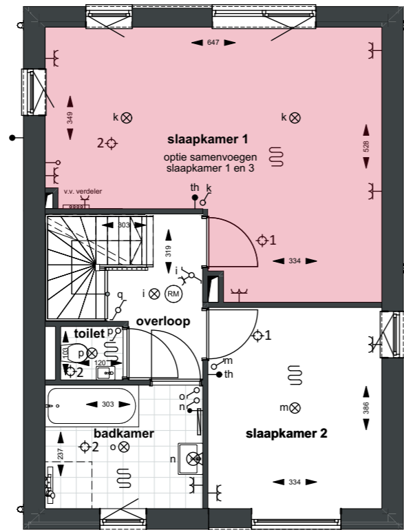
VERDIEPING
