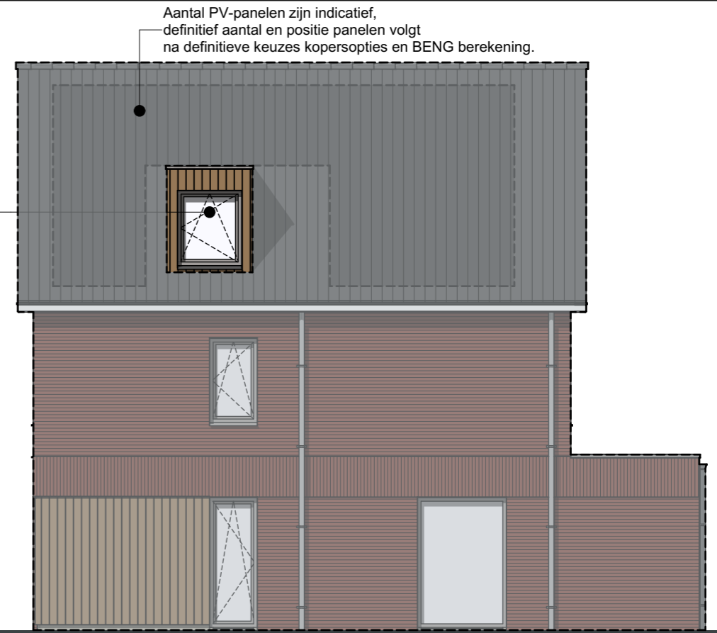
RECHTERGEVEL
