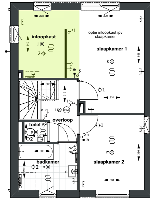
VERDIEPING
